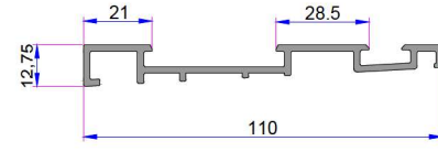
Alüminyum Eşik İkinci Kanat Ray 16025.451.5.2.0.0000 - 4,5 MT 16025.551.5.2.0.0000 - 4,5 MT 16025.651.5.2.0.0000 - 4,5 MT
