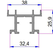
Kasa Üst Ray Alüminyum 16019.451.5.2.0.0000 - 4,5 MT 16019.551.5.2.0.0000 - 4,5 MT 16019.651.5.2.0.0000 - 4,5 MT
