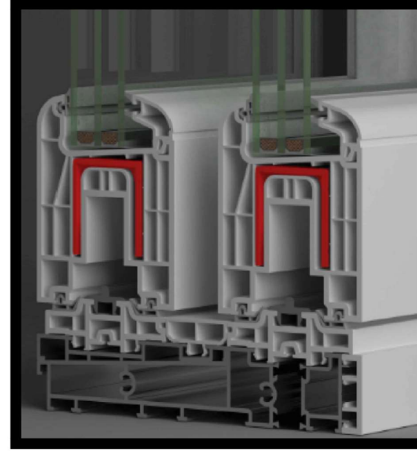
Hebeschiebe Orta Kanal Kapama P.A.930.6505.600
