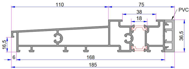
Hebeschiebe İç Kısmı PVC Isı Yalıtımlı Alm. Eşik Profili 16026.451.5.2.0.0000 - 4,5 MT 16026.551.5.2.0.0000 - 4,5 MT 16026.651.5.2.0.0000 - 4,5 MT
