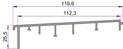
Hebeschiebe Alüminyum Eşik Kapama 16024.451.5.2.0.0000 - 4,5 MT 16024.551.5.2.0.0000 - 4,5 MT 16024.651.5.2.0.0000 - 4,5 MT
