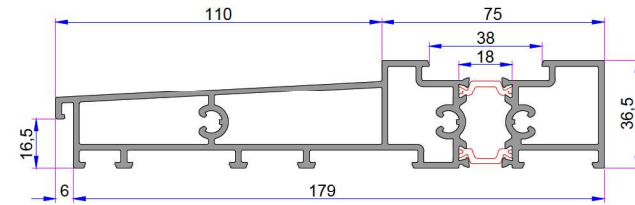
Hebeschiebe Isı Yalıtımlı Alm. Eşik Profili 16027.451.5.2.0.0000 - 4,5 MT 16027.551.5.2.0.0000 - 4,5 MT 16027.651.5.2.0.0000 - 4,5 MT
